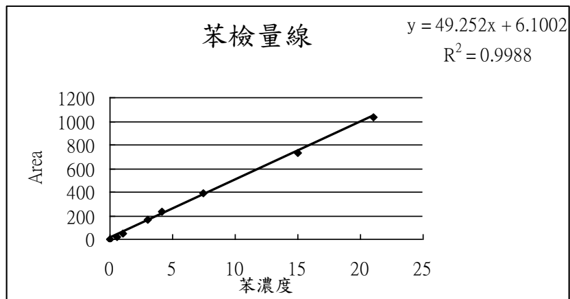
圖 3.2 苯檢量線
